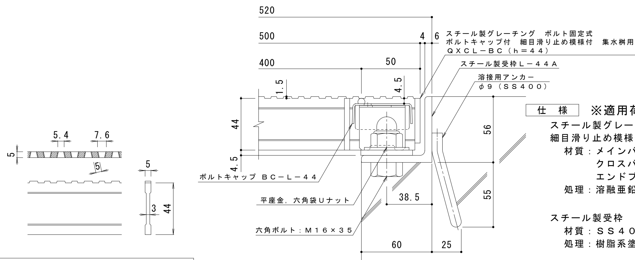
D I - 4 4 バ一形状詳細 S = 1 : 2
