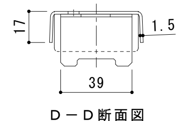
ボルトキャップBC-L詳細図
