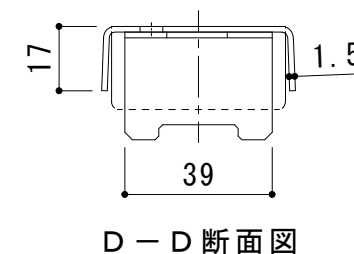
ボルトキャップBC-L詳細図
