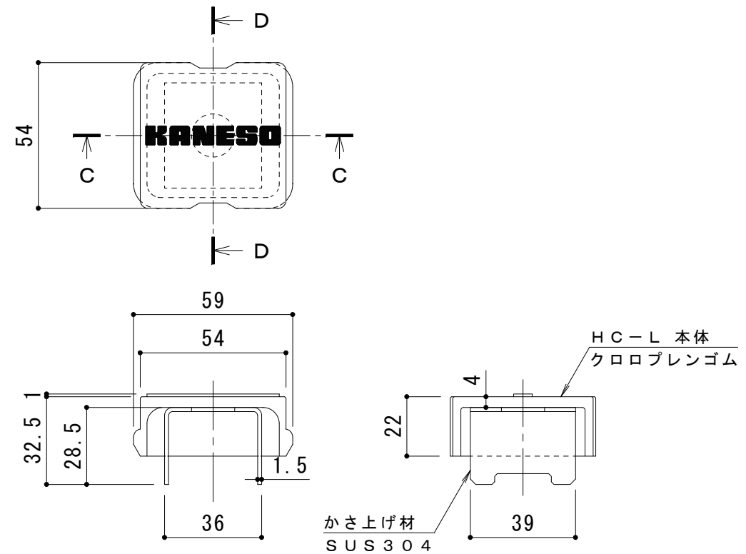
C - C 断面図 D - D 断面図
