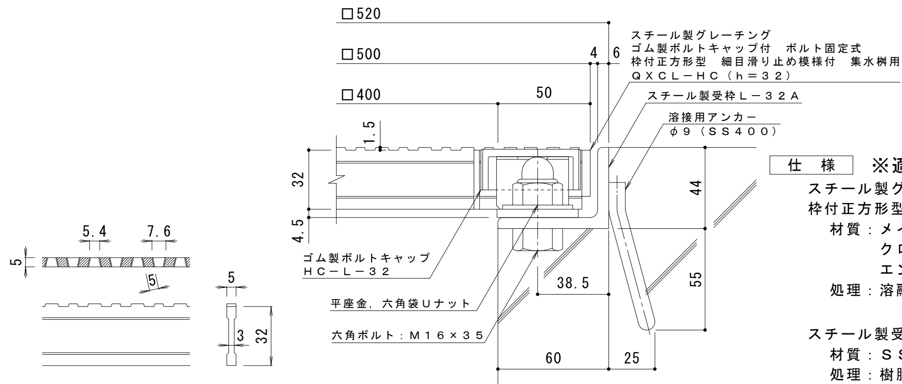
DI-32 バー形状詳細 S = 1 : 2
