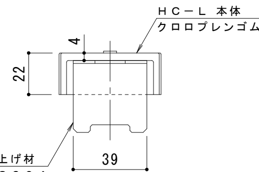
D - D 断面図
