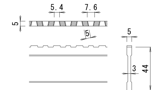
DI-44 バー形状詳細 S=1:2
