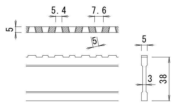
DI-38 バー形状詳細 S=1:2
