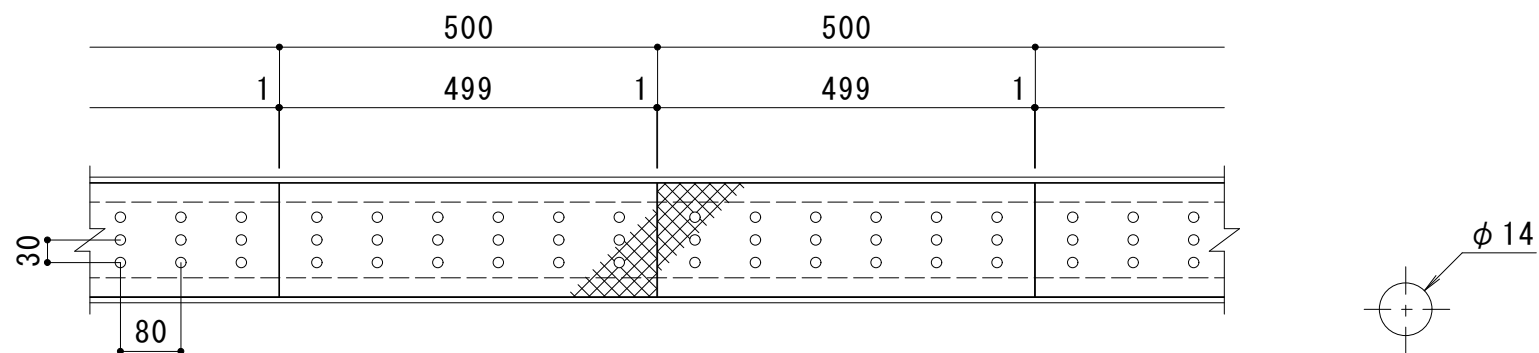
平面詳細図 S = 1 : 10
