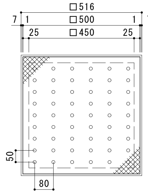
排水穴詳細 S = 1 : 2
