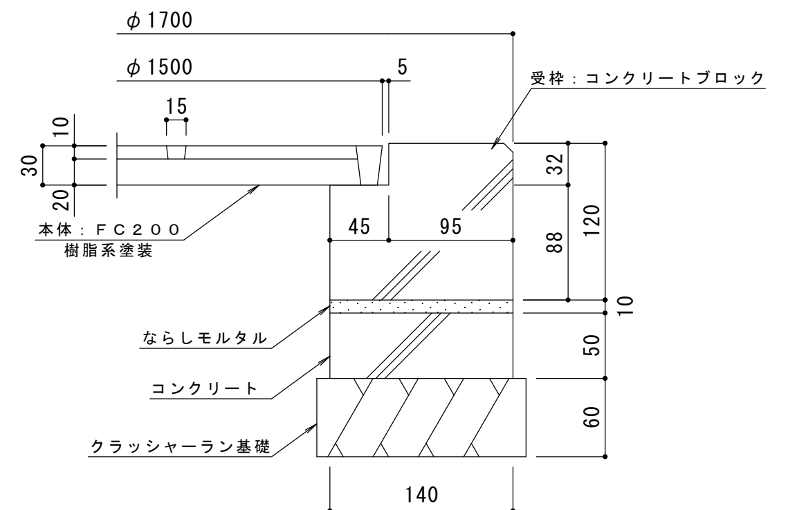
納まり詳細図 S = 1 : 4
