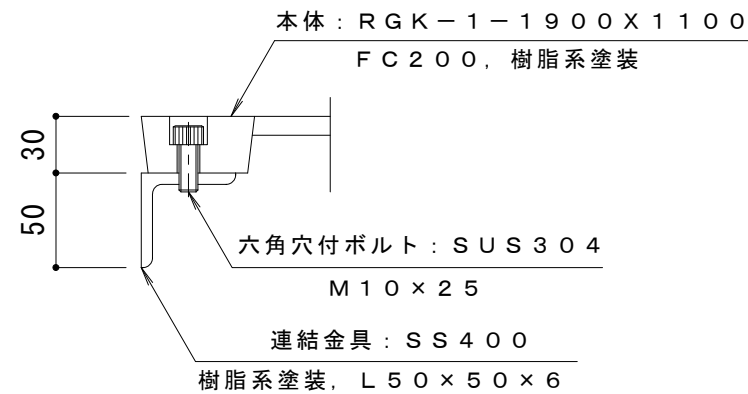
連結部詳細 S = 1 : 4 ※本体は4分割です。
