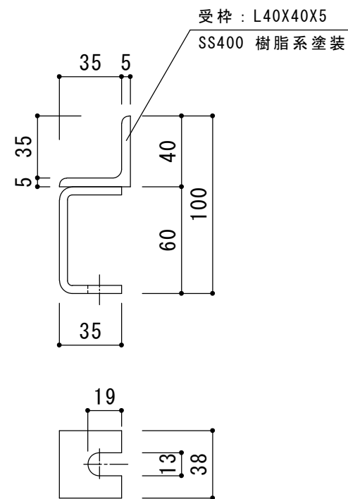
断面詳細図 S = 1 : 3
