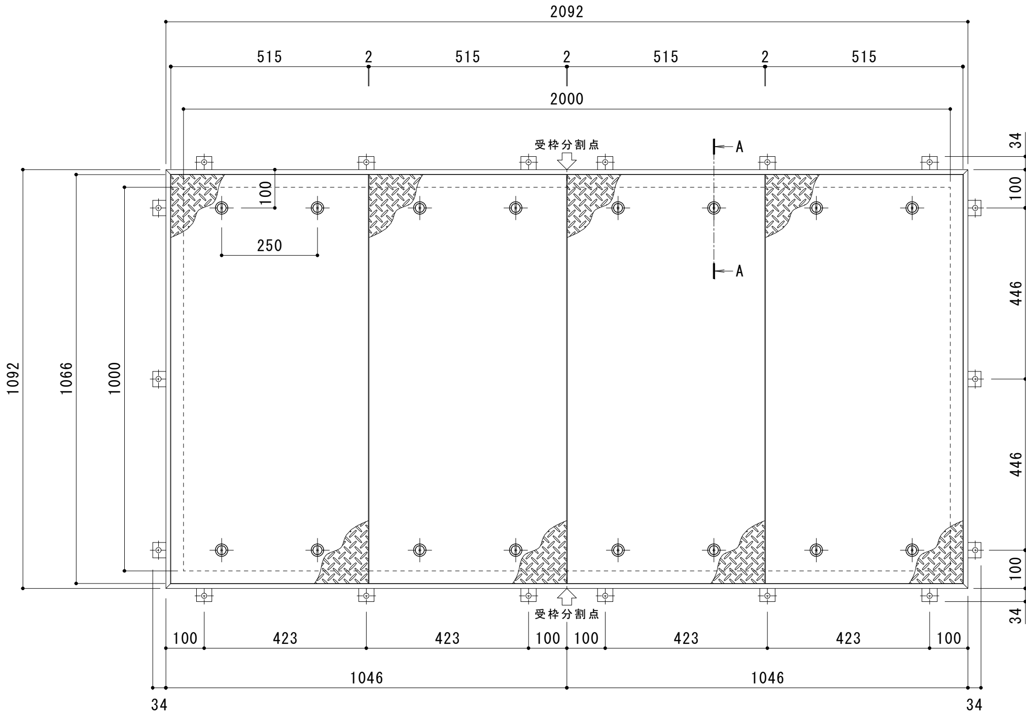
平面詳細図 S = 1 : 1 0
