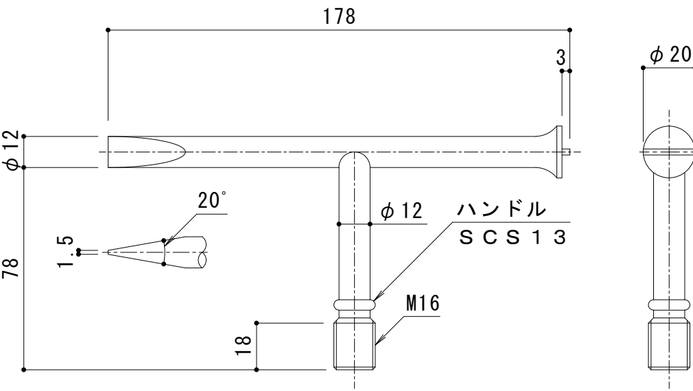
別売部品 開閉ハンドル詳細図 S = 1 : 2 K-1b型（4本／組）
