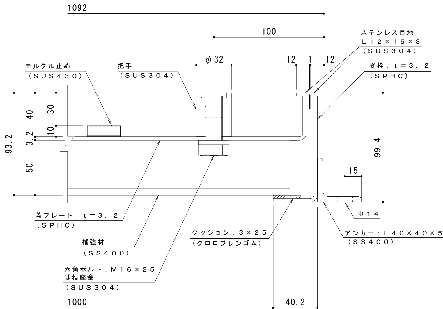
A-A断面詳細図 S = 1 : 2 表面処理：下塗り＋焼付塗装（但し目地、把手、クッション材を除く）
