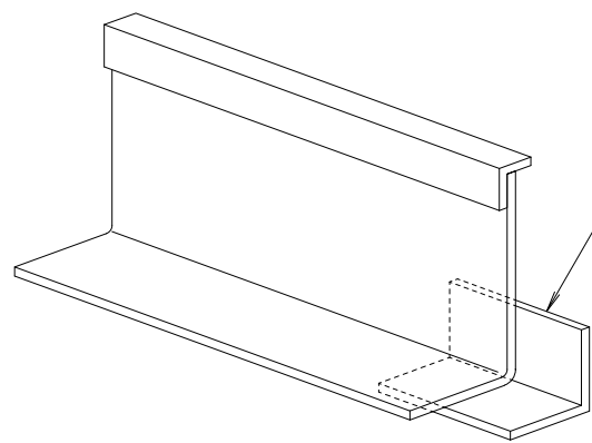
受枠連結部詳細図
