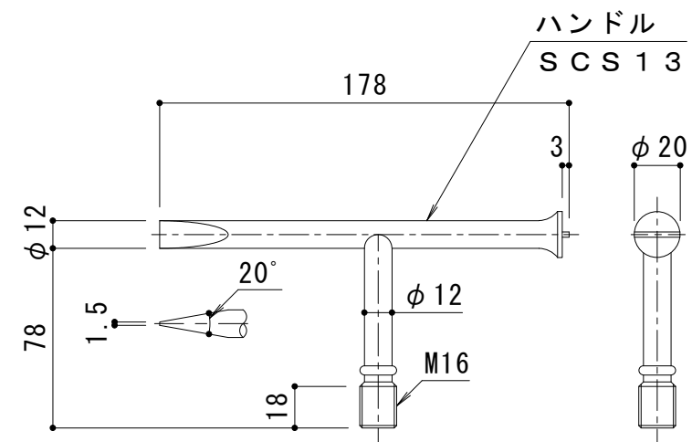
別売部品 開閉ハンドル詳細図 S = 1 : 3
