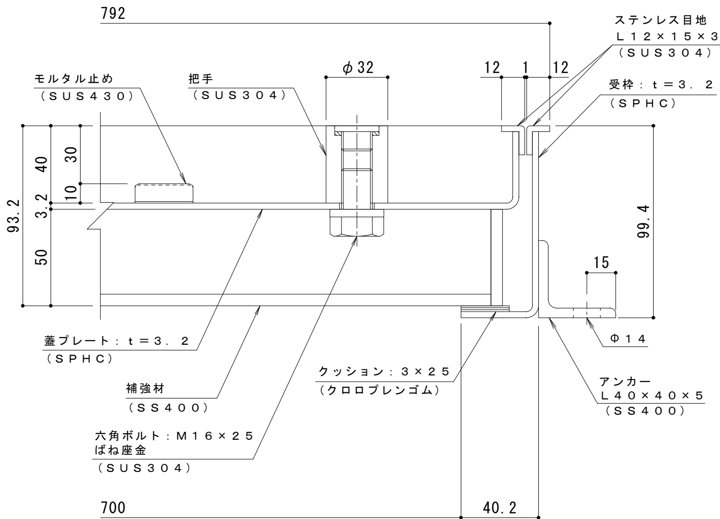
A-A断面詳細図 S = 1 : 2
