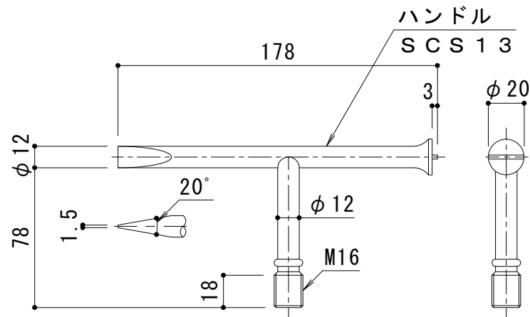
別売部品 開閉ハンドル詳細図 S = 1 : 3
