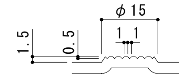
滑り止め詳細 S = 1 : 1
