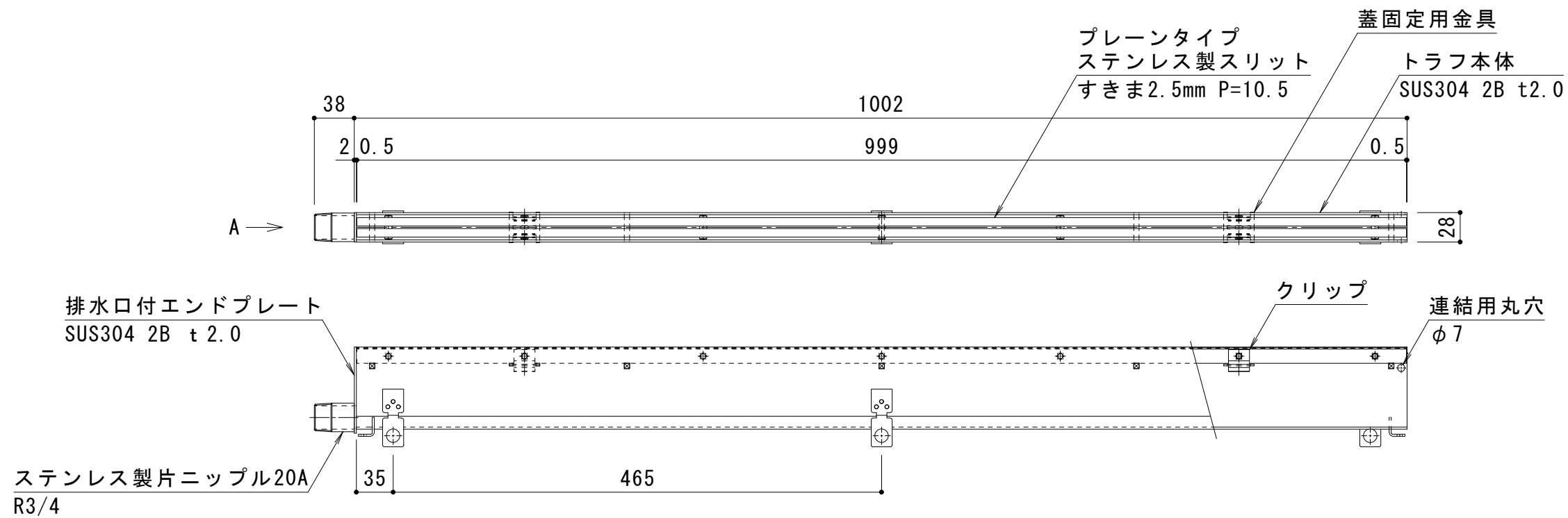
製品詳細図 S = 1 : 5
