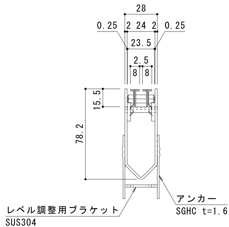
A 矢視図 S = 1 : 2
