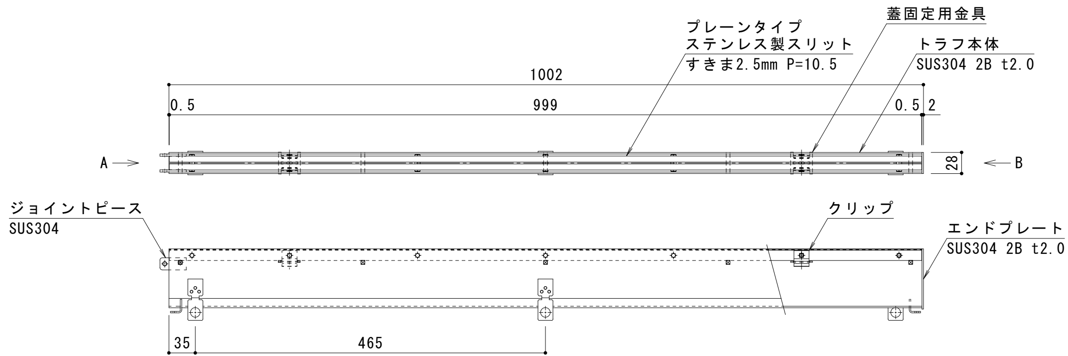
製品詳細図 S = 1 : 5
