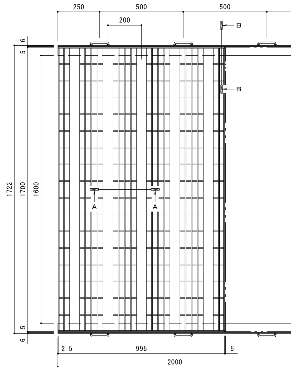
平面図 S = 1 : 1 0
