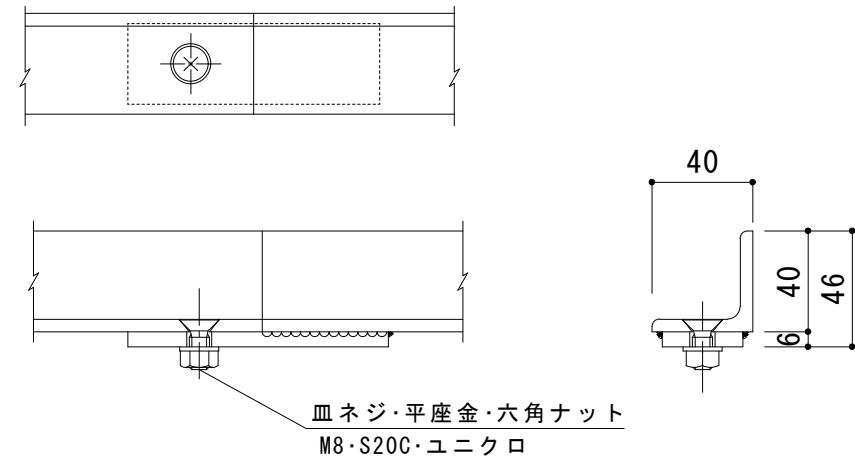
接続部詳細図 S = 1 : 3
