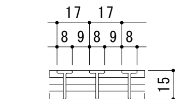
A断面図 S = 1 : 2
