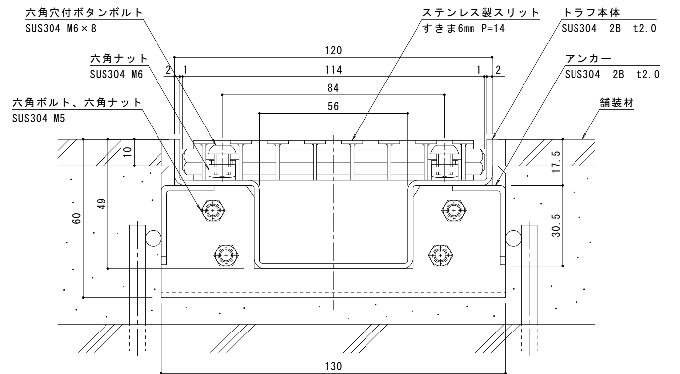
断面納まり図 S = 1 : 1
