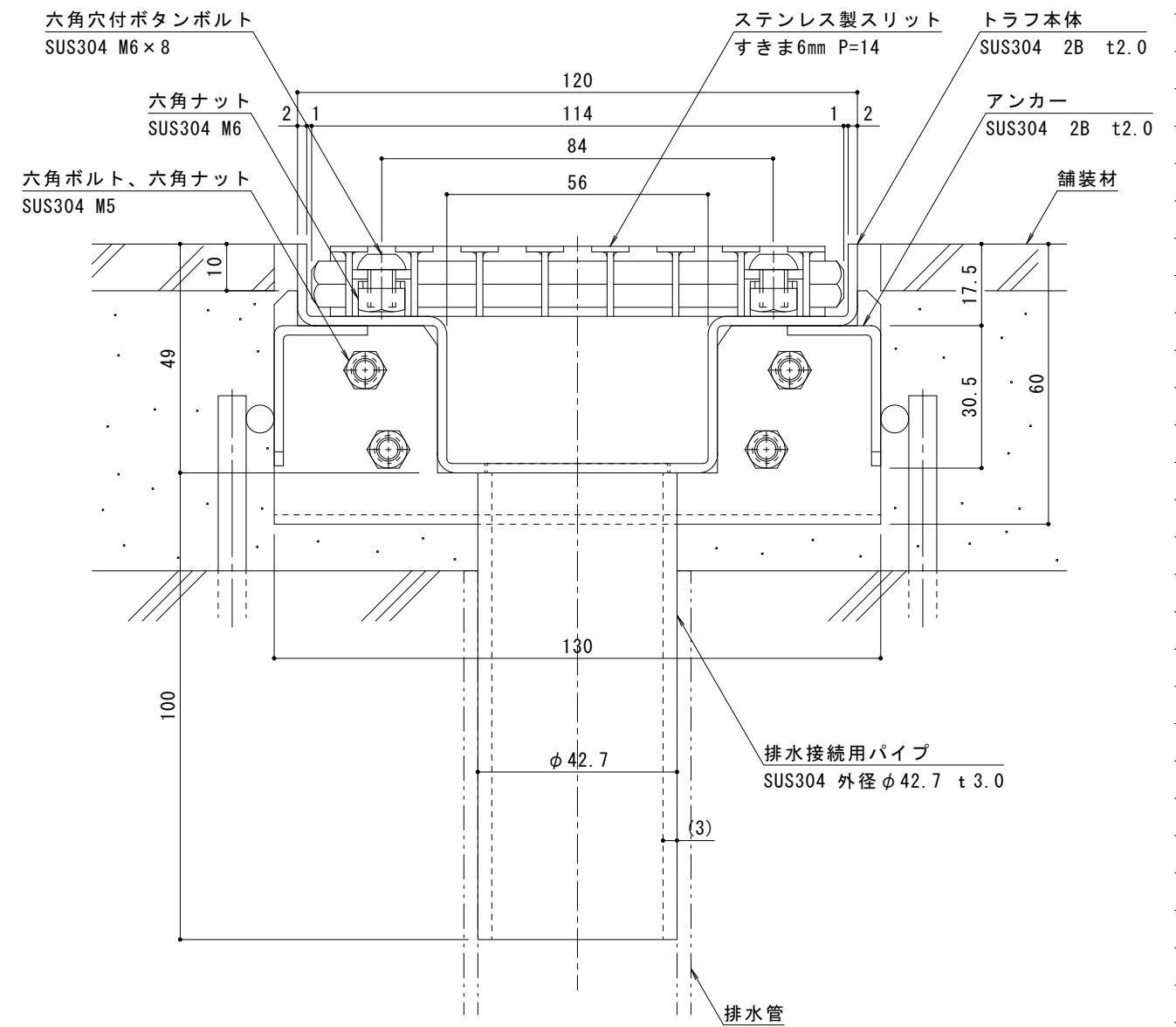
断面納まり図 S = 1 : 1
