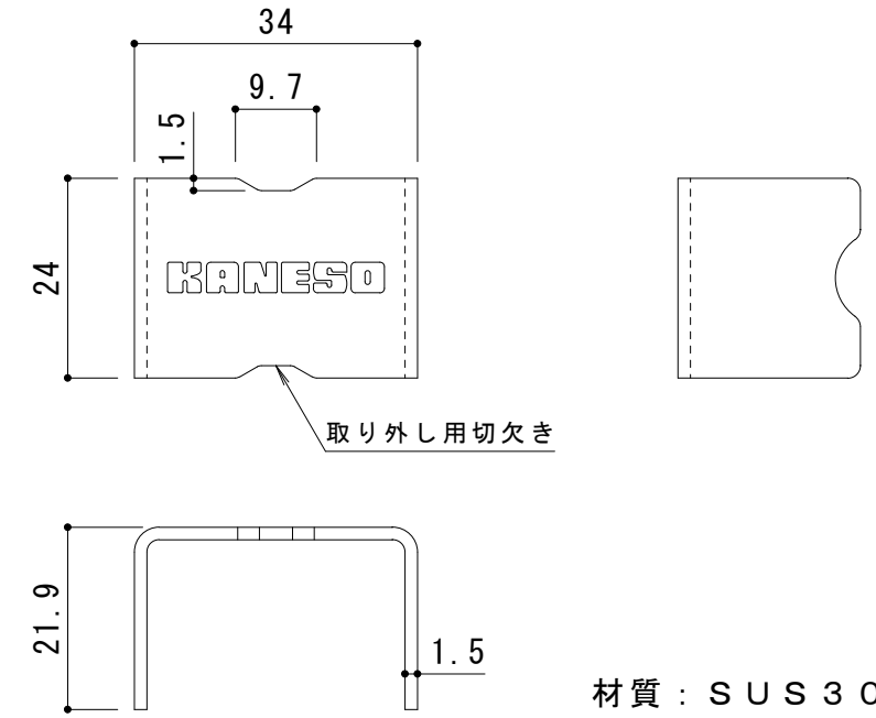
ボルトキャップDC-3-25詳細図 S = 1 : 1
