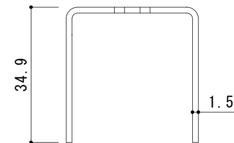
ボルトキャップ DC-3-38 詳細図 S = 1 : 1
