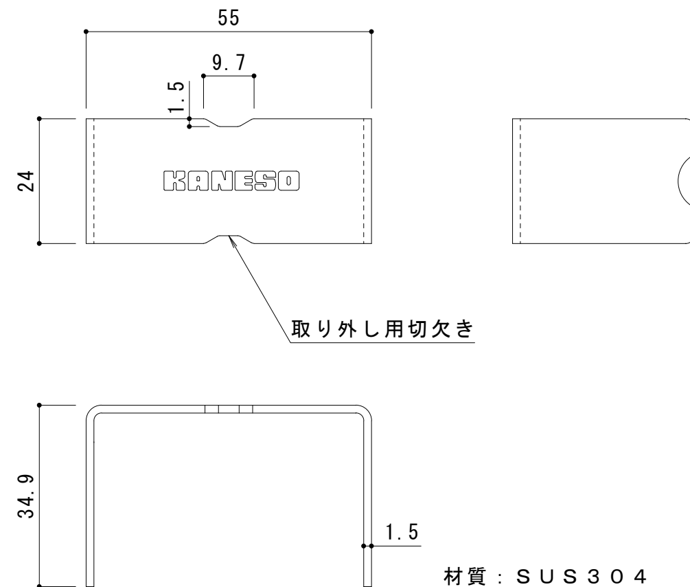
ボルトキャップDC-1-38詳細図 S = 1 : 1
