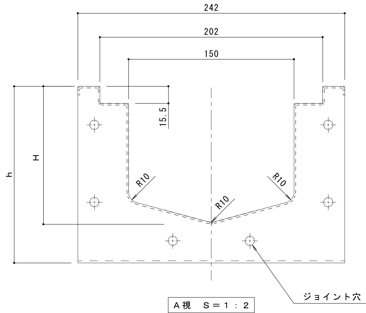
ジョイント穴詳細
