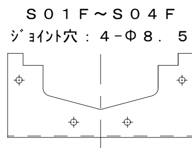
ジョイント穴詳細
