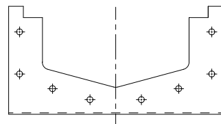
V05~V11 ジョイント穴: 8-Φ8.5
