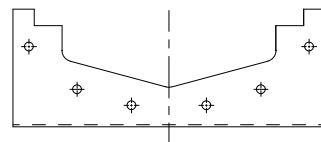
V01~V04 ジョイント穴: 6-Φ8.5
