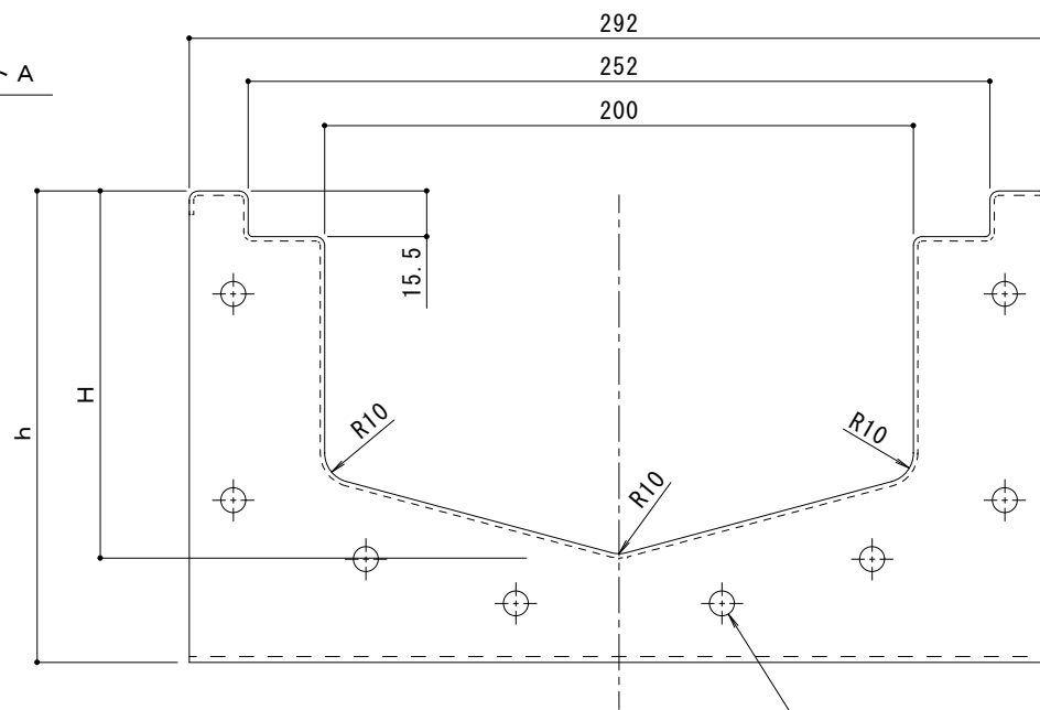
A視 S=1:2
