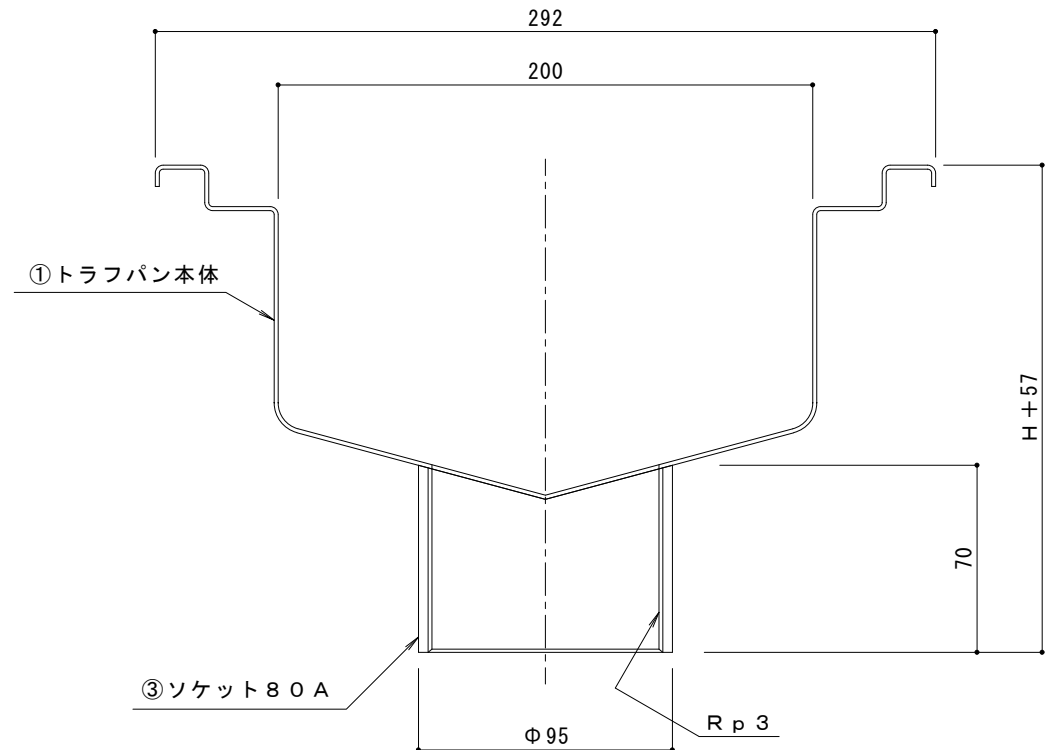
C-C断面 S=1:2
