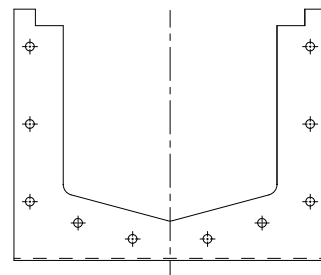
V12~V18 ジョイント穴: 10-Φ8.5
