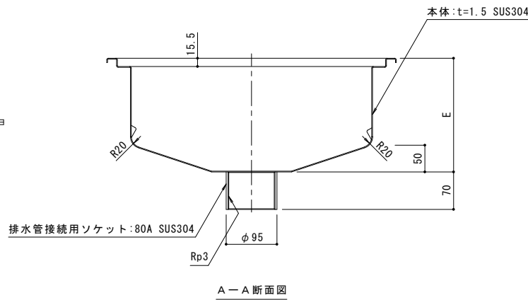
納まり図（埋設）
