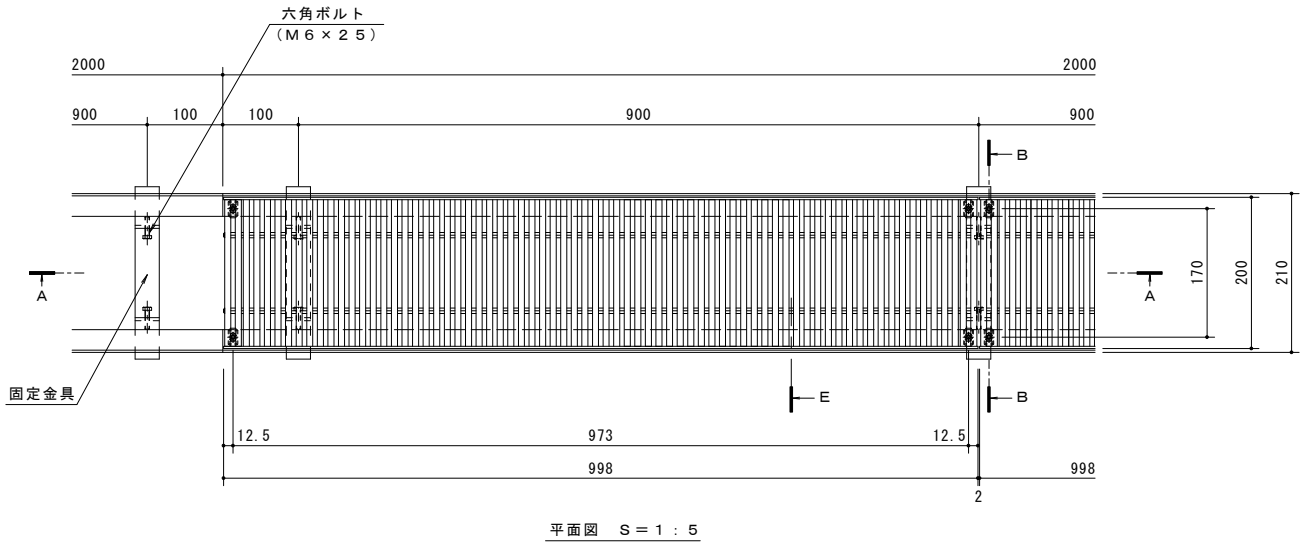
平面図 S = 1 : 5
