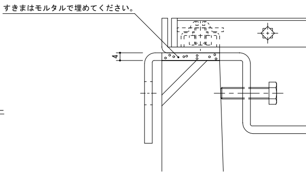
E断面詳細図 S = 1 : 1
