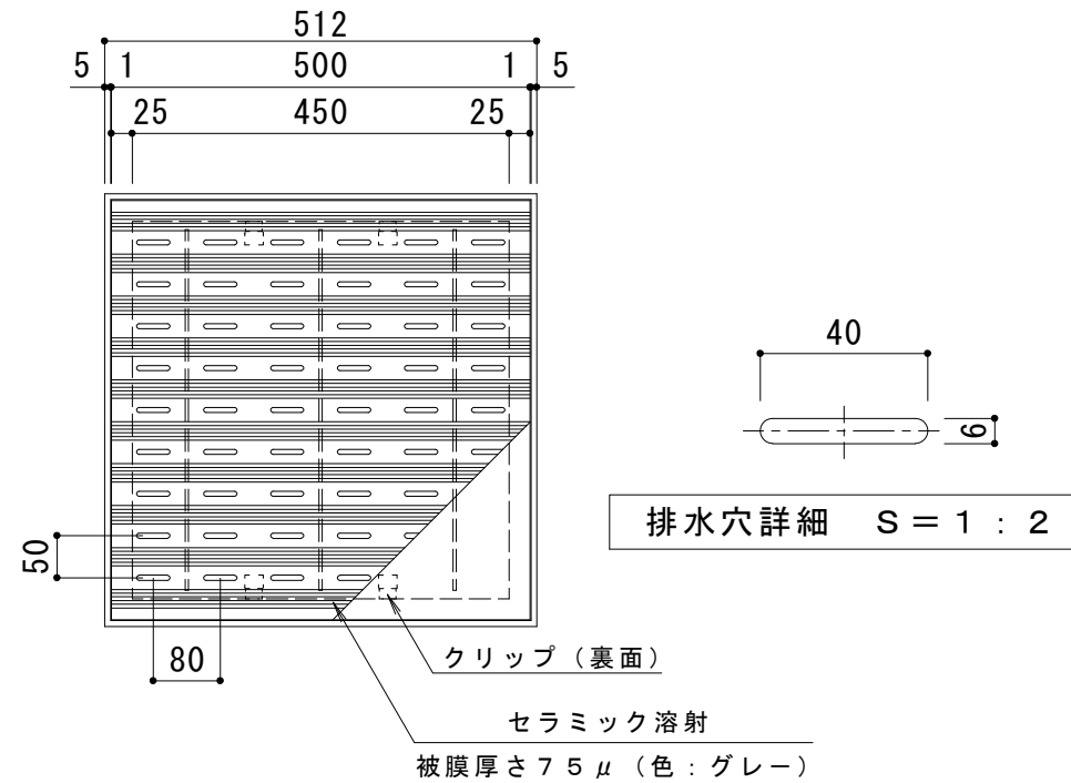
平面詳細図 S = 1 : 1 0
