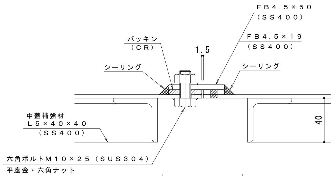
中蓋連結部詳細 2分割
