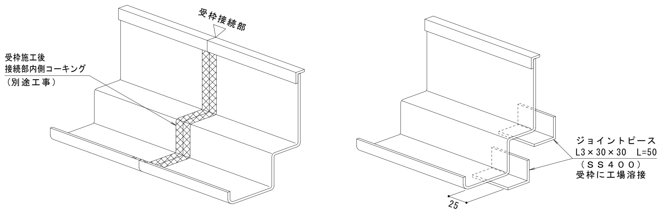
受枠接続部詳細 2分割
