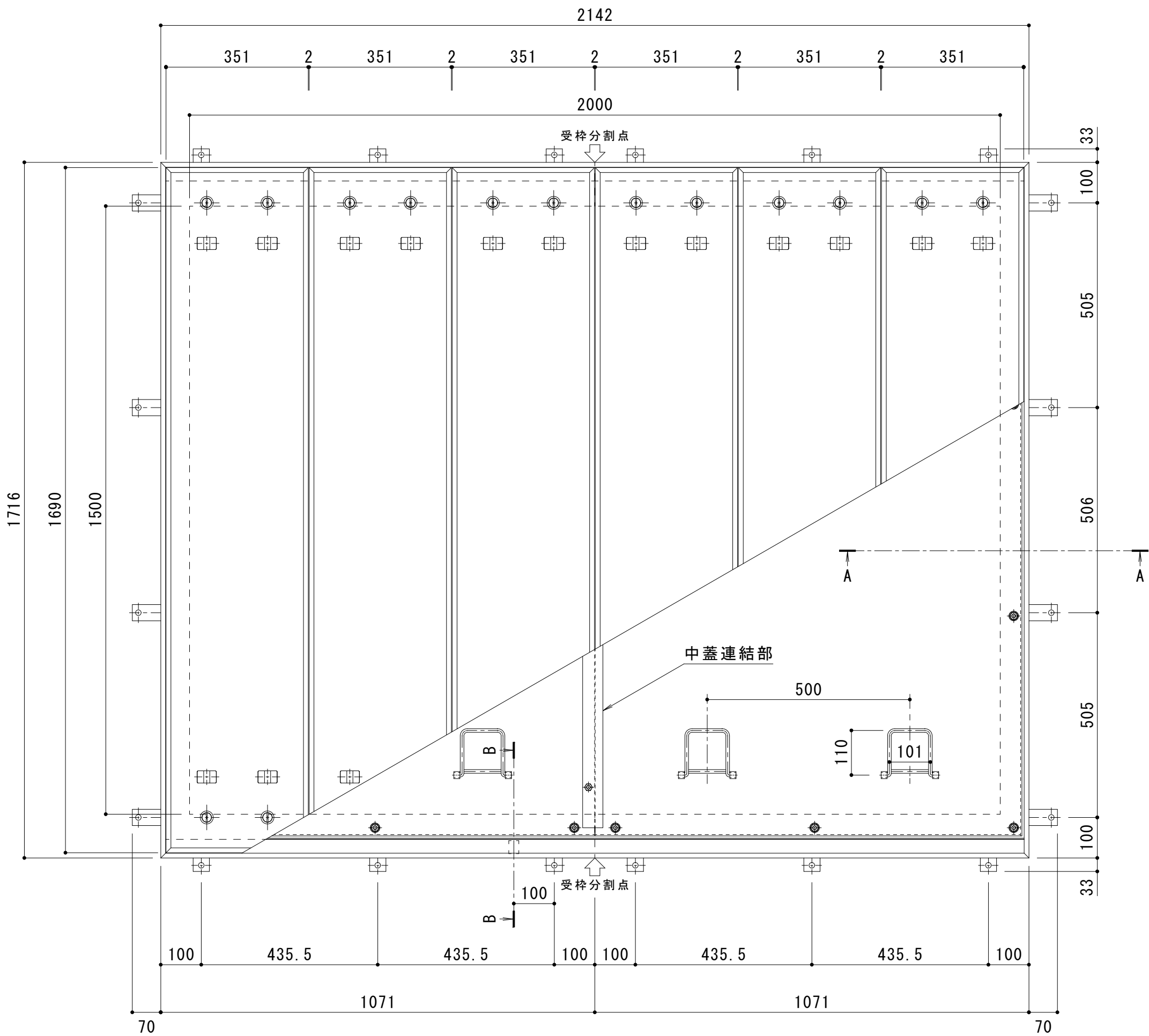
平面詳細図 S = 1 : 1.0
