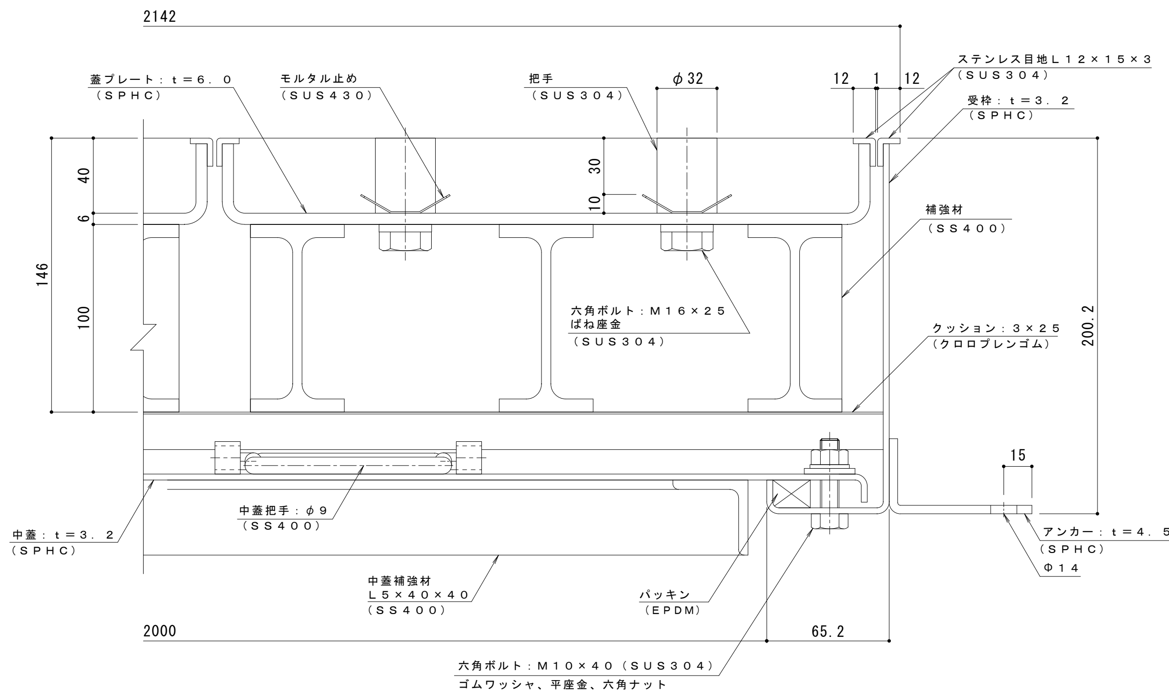
A-A断面詳細図 S = 1 : 2
