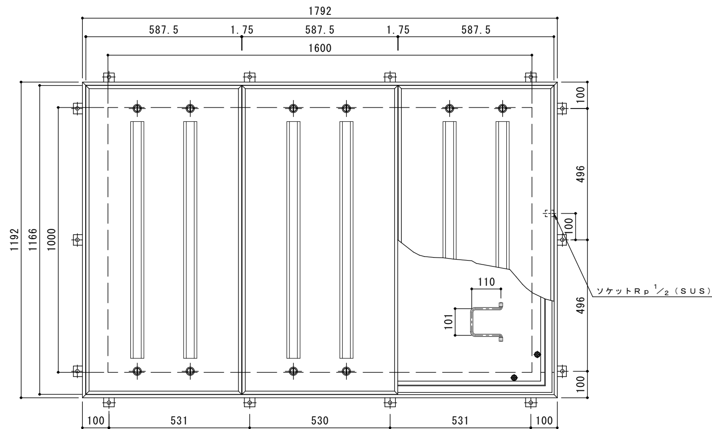
平面詳細図 S = 1 : 10
