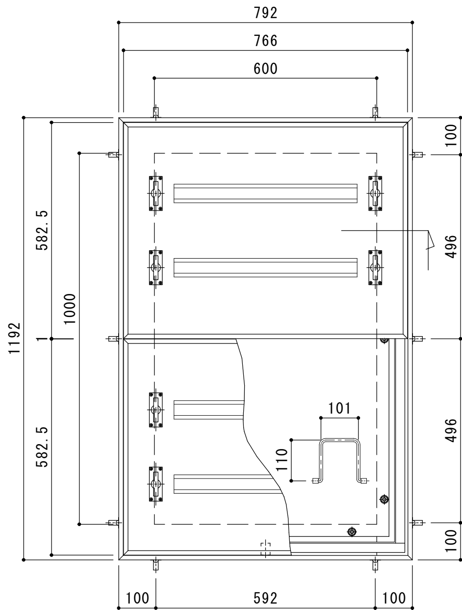
平面詳細図 S = 1 : 1 0
