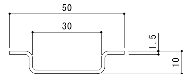
モルタル止め 補強材詳細図 S = 1 : 1
