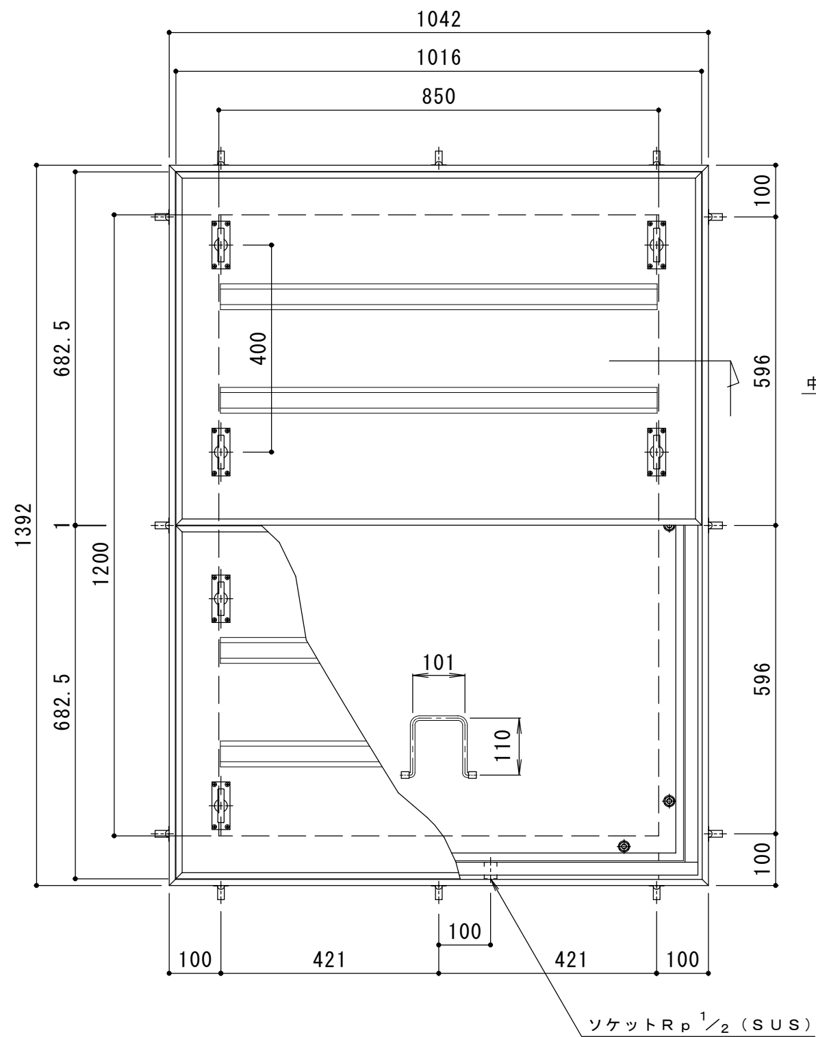
平面詳細図 S = 1 : 1 0
