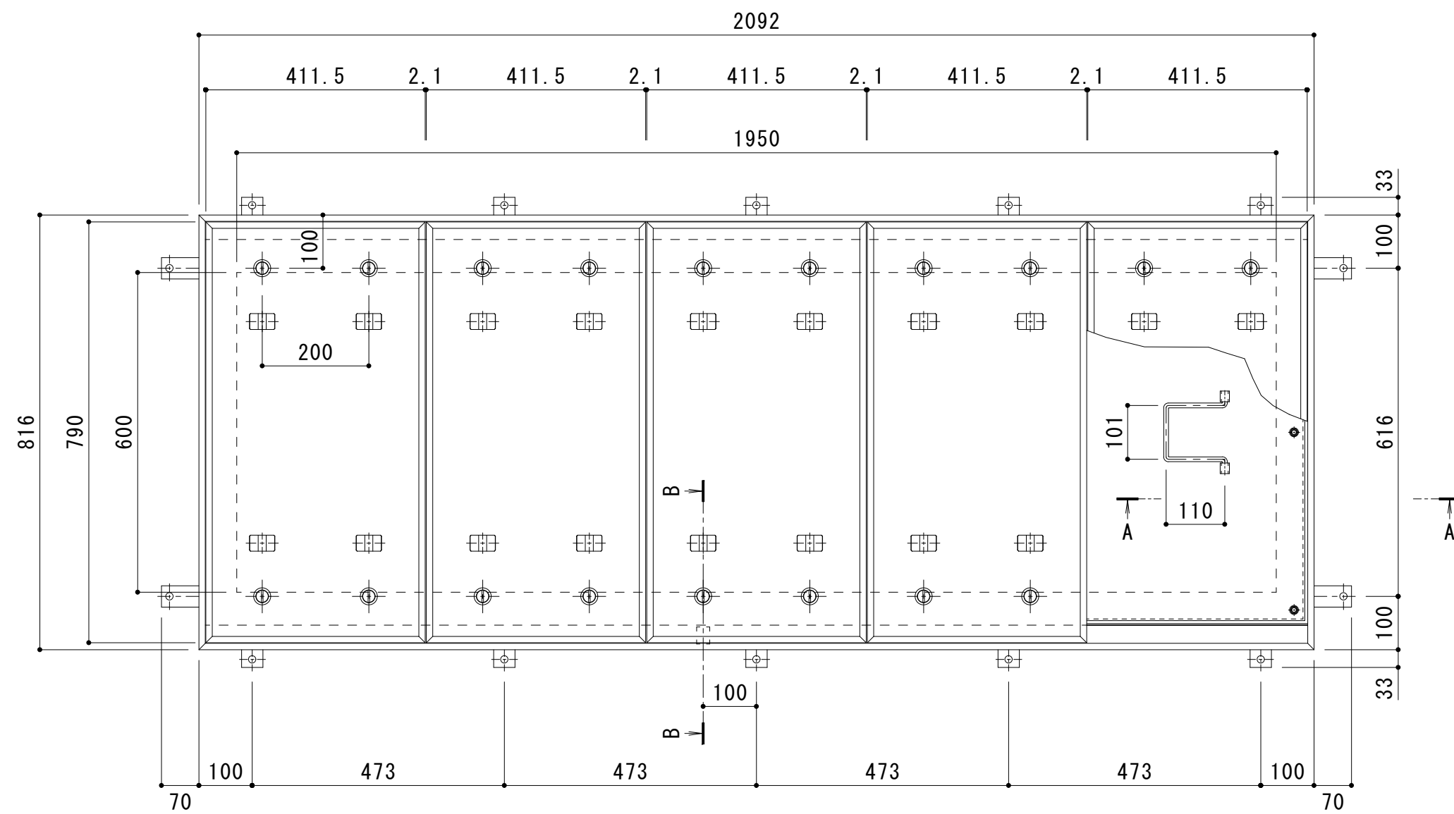
平面詳細図 S = 1 : 10
