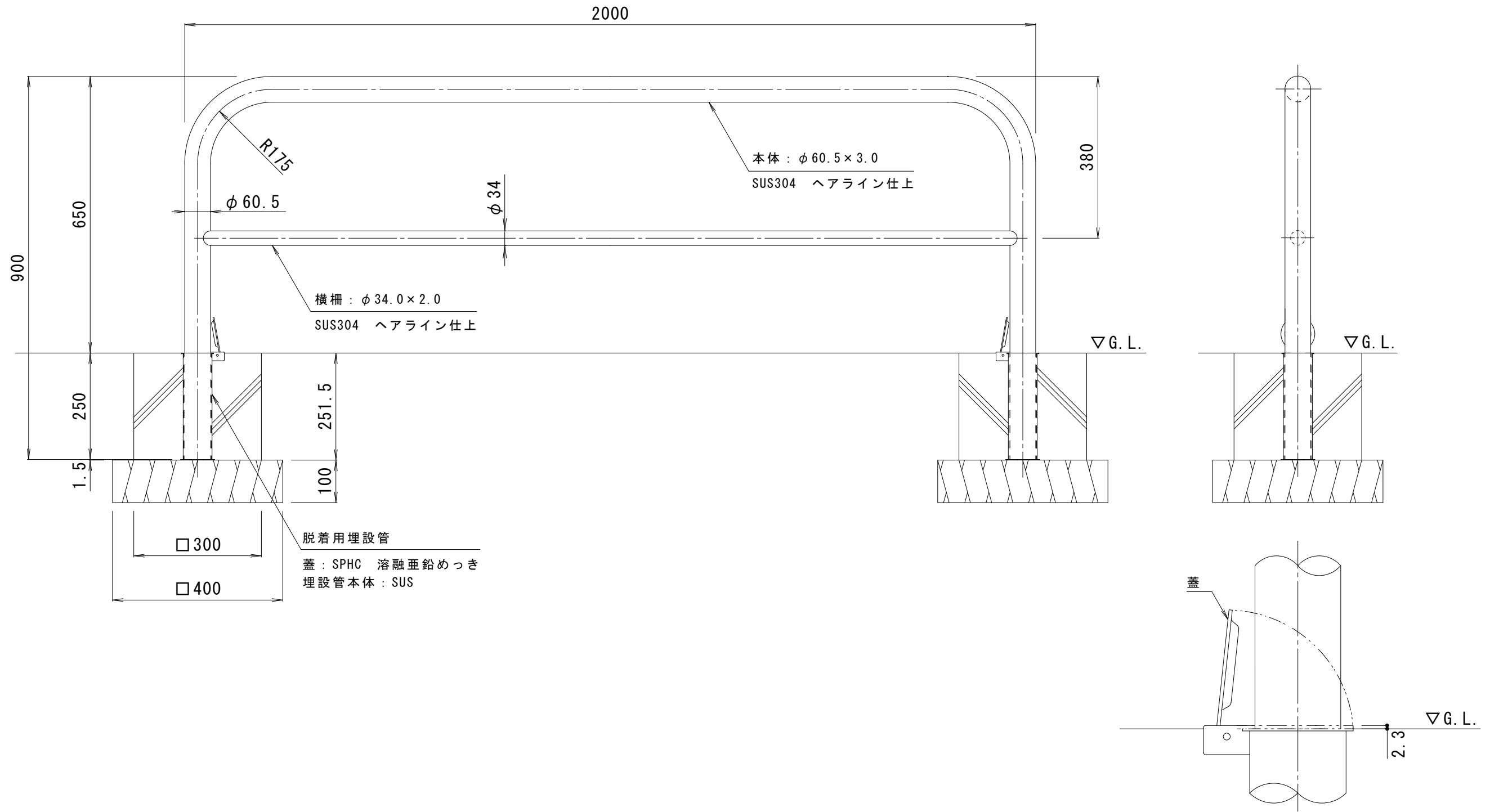
埋設管蓋部詳細図 S = 1 : 3
