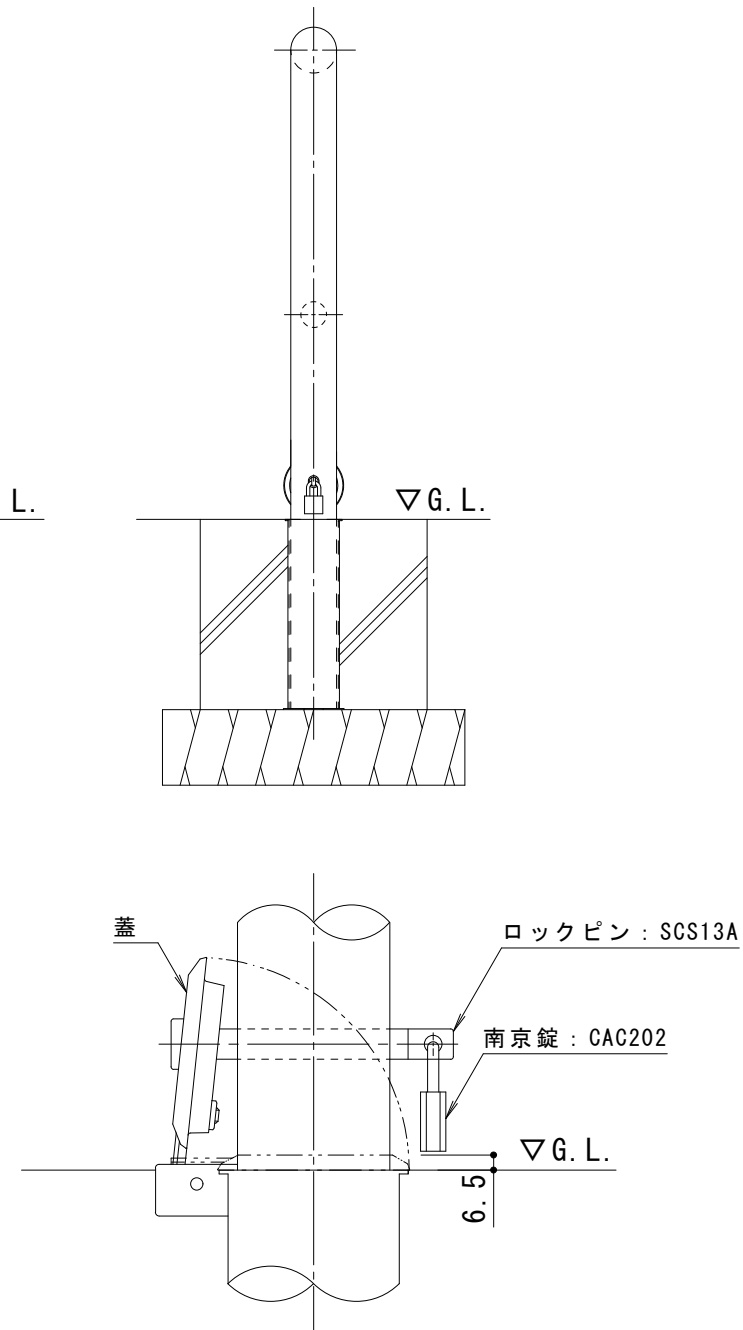
南京錠部詳細図 S = 1 : 3
