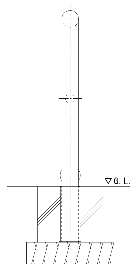
埋設管蓋部詳細図 S = 1 : 3
