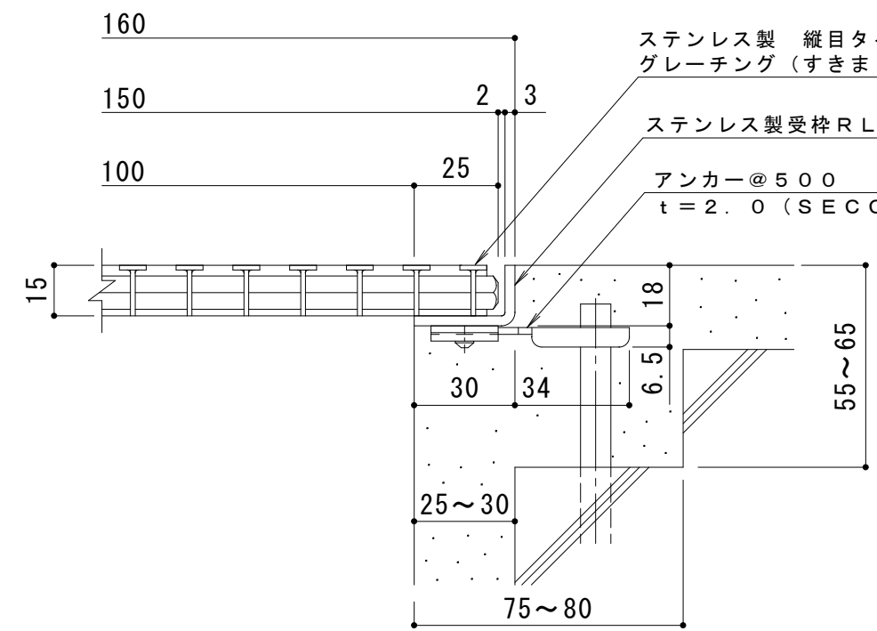
A断面詳細図 S = 1 : 2
