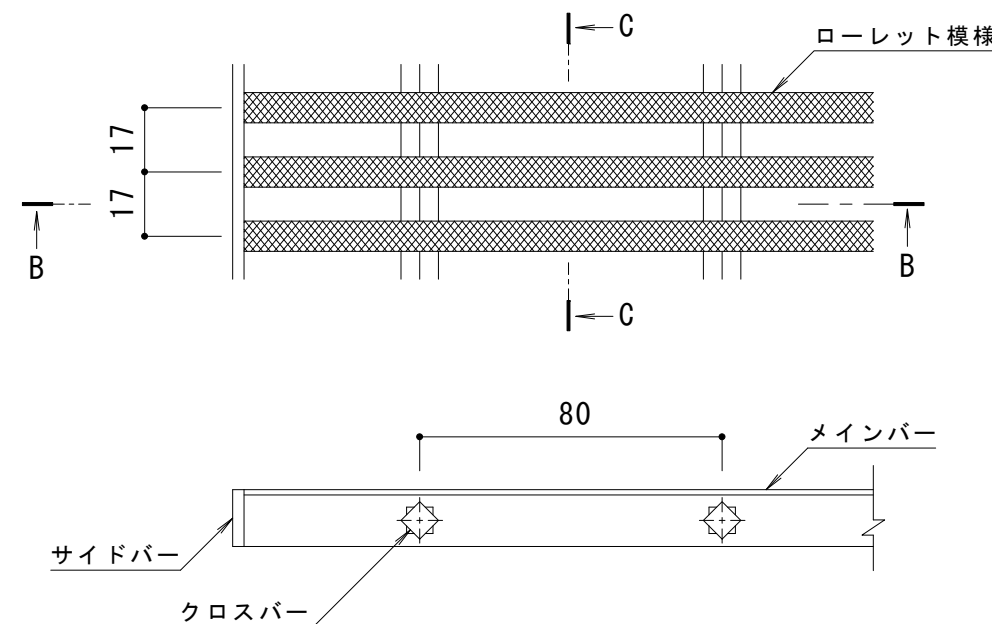
B-B断面図
