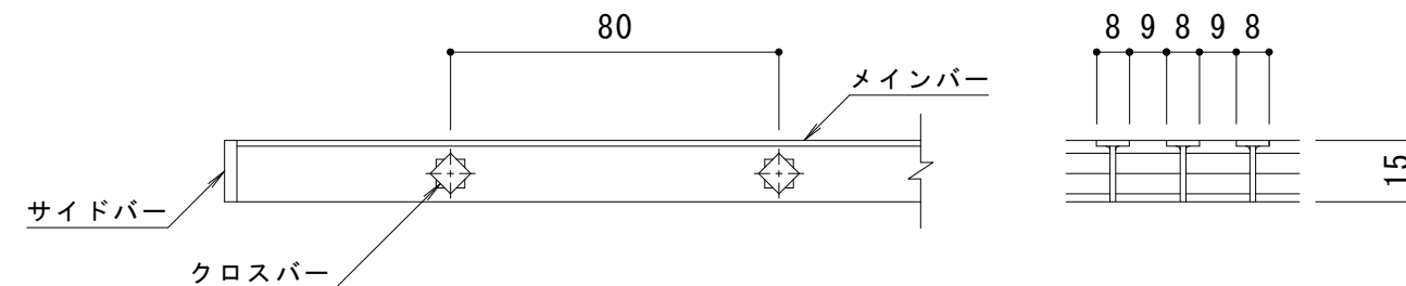
B-B断面図
