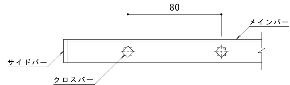
B-B断面図
