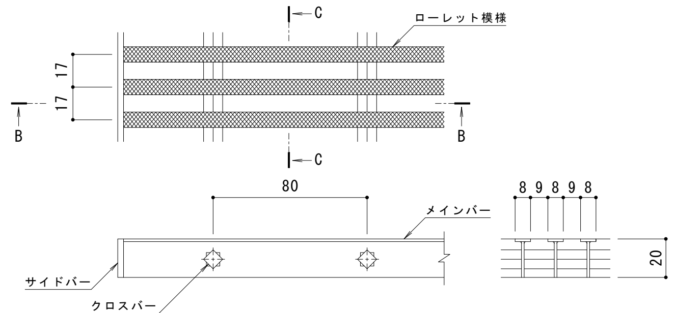
B-B断面図
