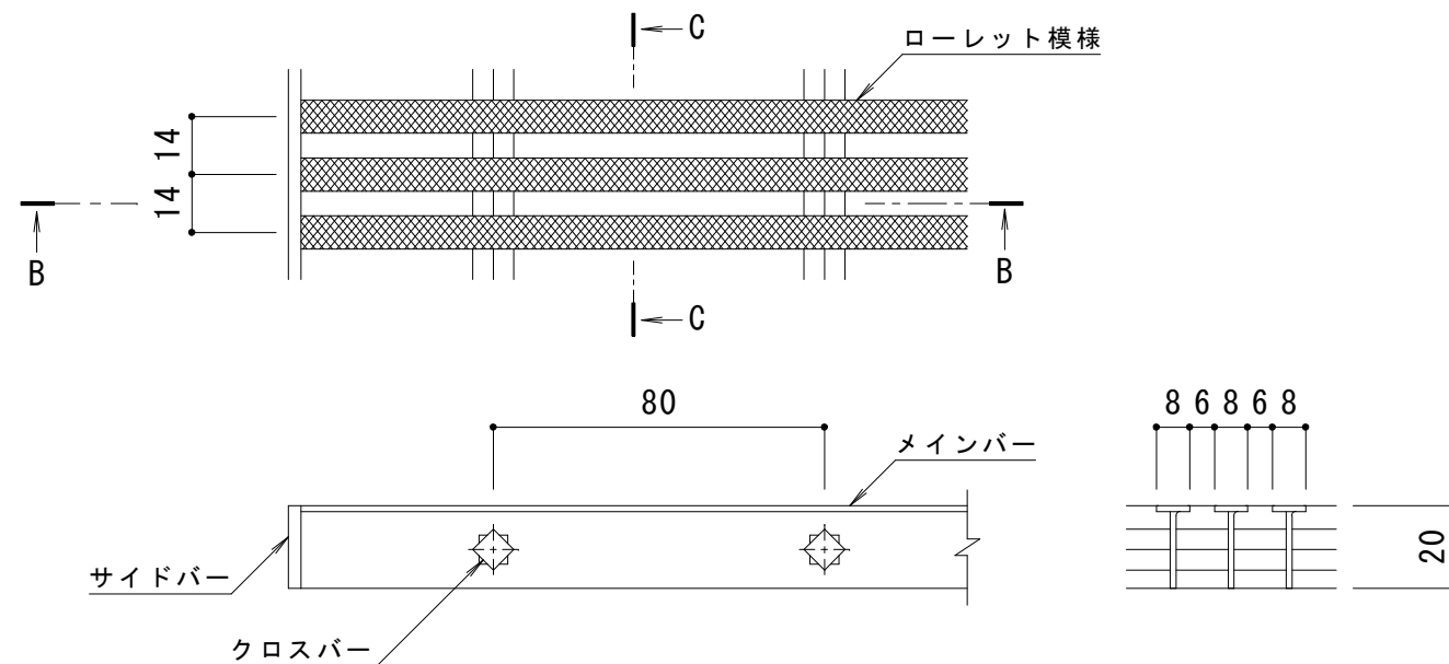
B-B断面図
