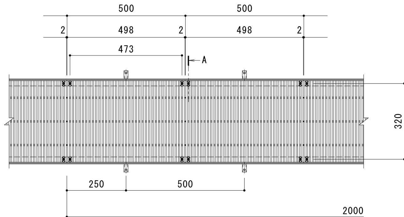
平面詳細図 S = 1 : 1 0
