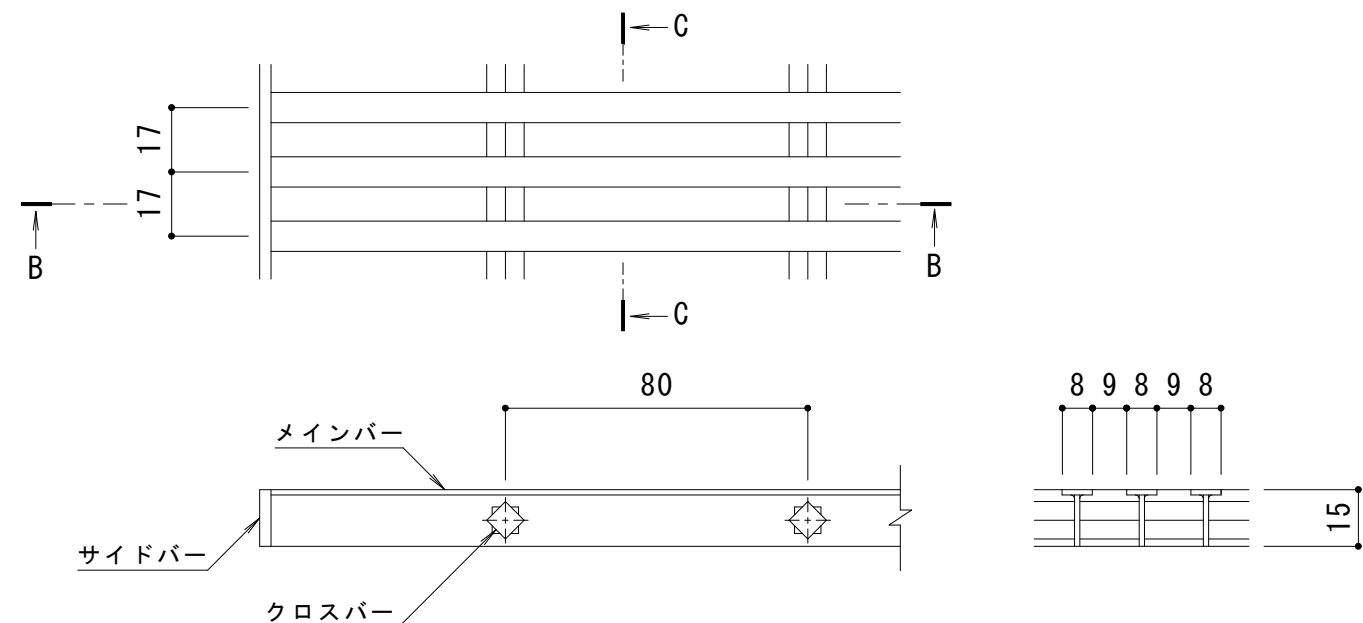
B-B断面图
